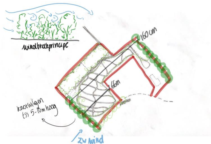
Figuur 4.10. In het noordwesten voorziet het huidige en te herbebossen bos de functie van windkering, net als de bestaande bomenrij in het zuidoosten. In het noordoosten en zuidwesten voorziet dit ontwerpvoorstel knotwilgen, aangepast aan de natte ondergrond. Deze wilgen kunnen voorzien in brandhout voor de kampeers of in wilgentenen voor vlechtworkshops (© HOGENT – Landschaps- en tuinarchitectuur – Workshop Voedselbos: Ameys Gaëtaan, Bruggeman Jeroen, Guerzoni-Verschuere Colomba, Moens Ellen, Moernaut Lisa en Ostyn Brennin).
